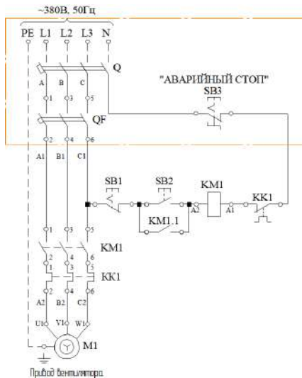
Схема подключения пускателя с катушкой на 220 В
