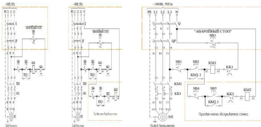
Схема подключения пускателя с катушкой на 220 В
