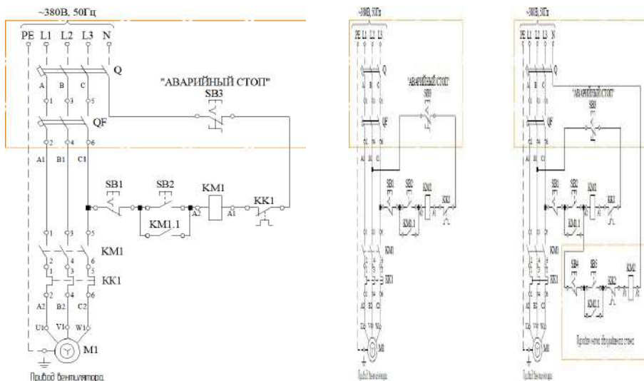
Схема подключения пускателя с катушкой на 220 В
